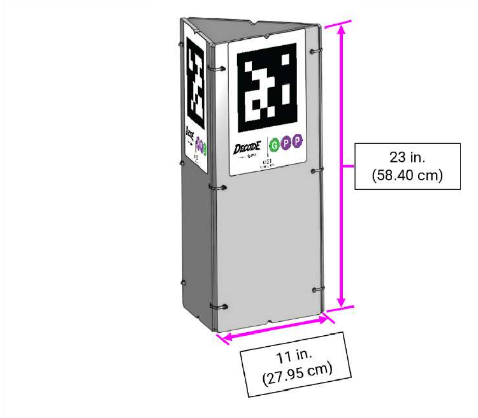
圖 9-7：方尖碑尺寸
