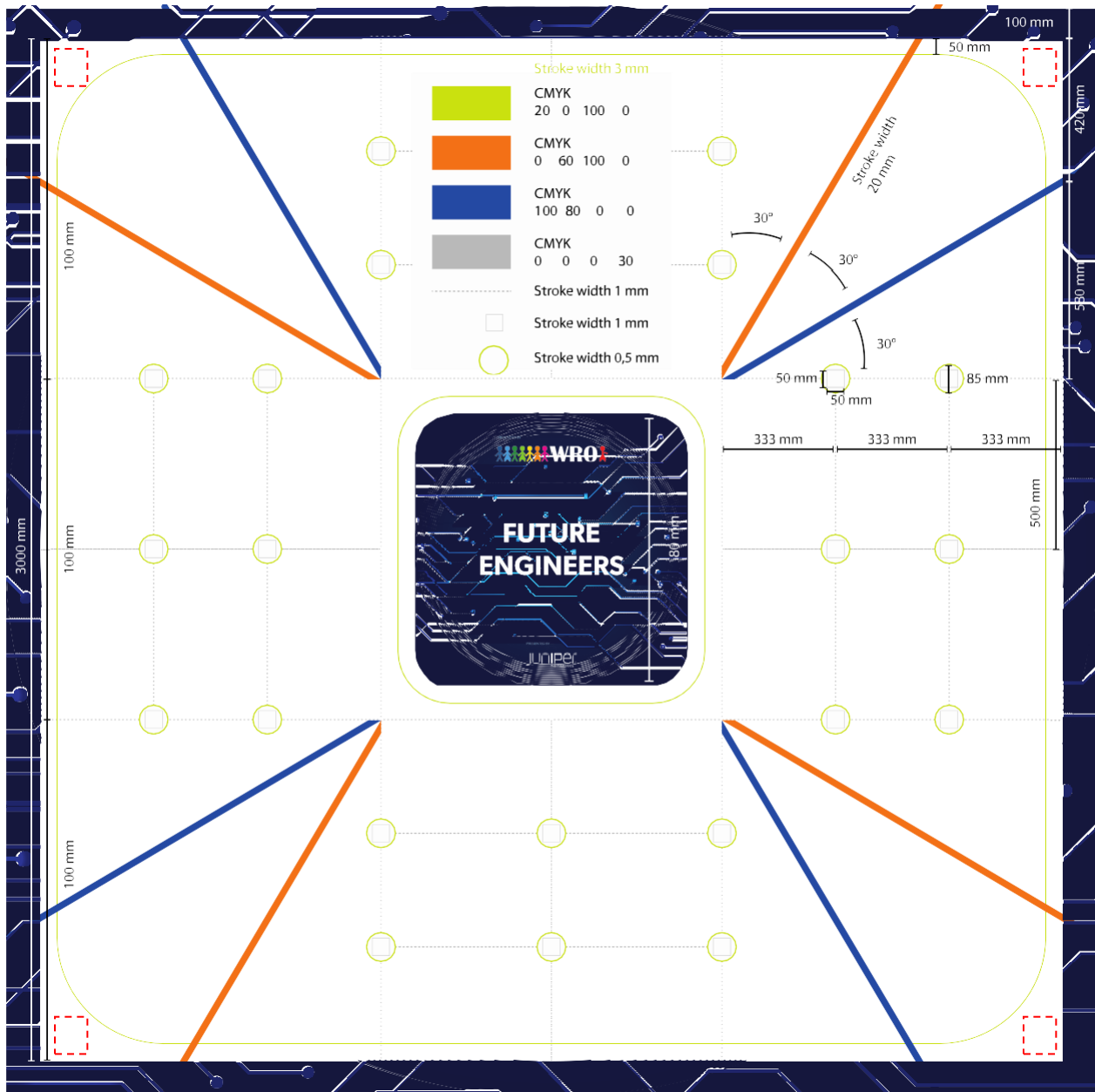
圖 12. 場地底圖尺寸 (紅色虛線區處會印製贊助單位)
