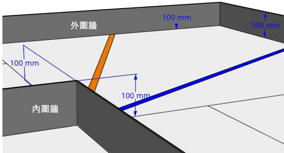
圖 13. 內圍牆及外圍牆的高度尺寸
