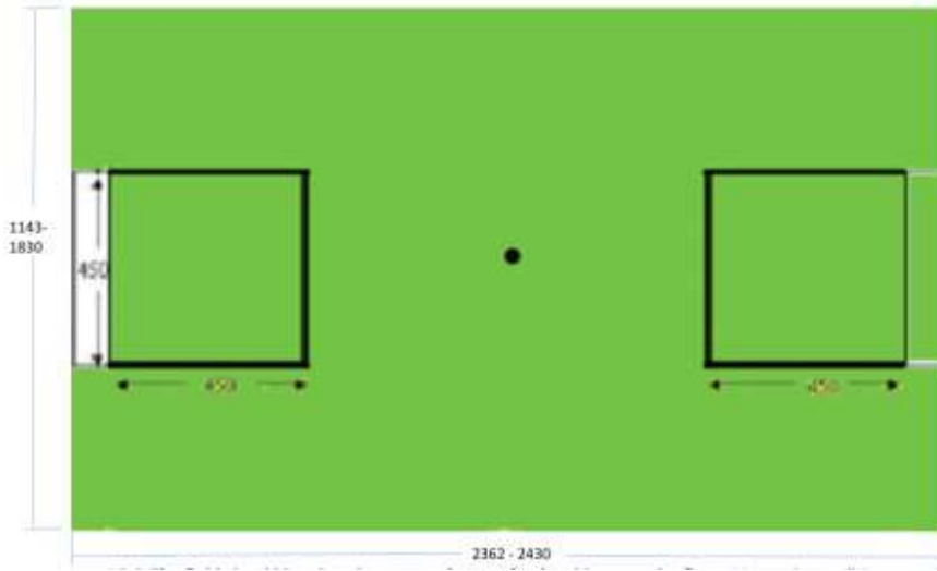
足球場地尺寸圖
